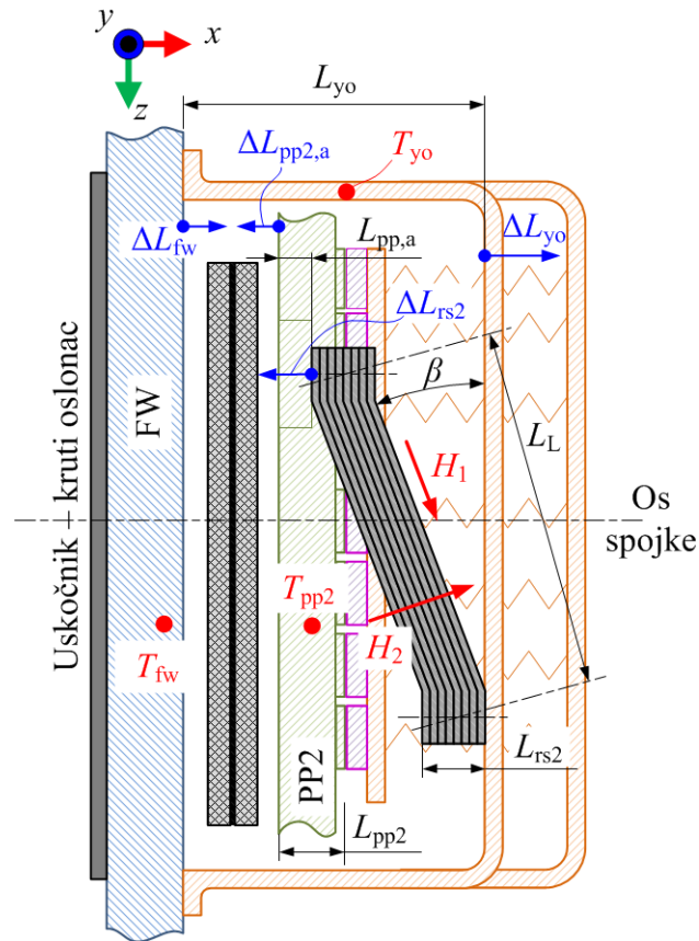
Slika 7-7: Ilustracija toplinskog širenja za otvorenu spojku
