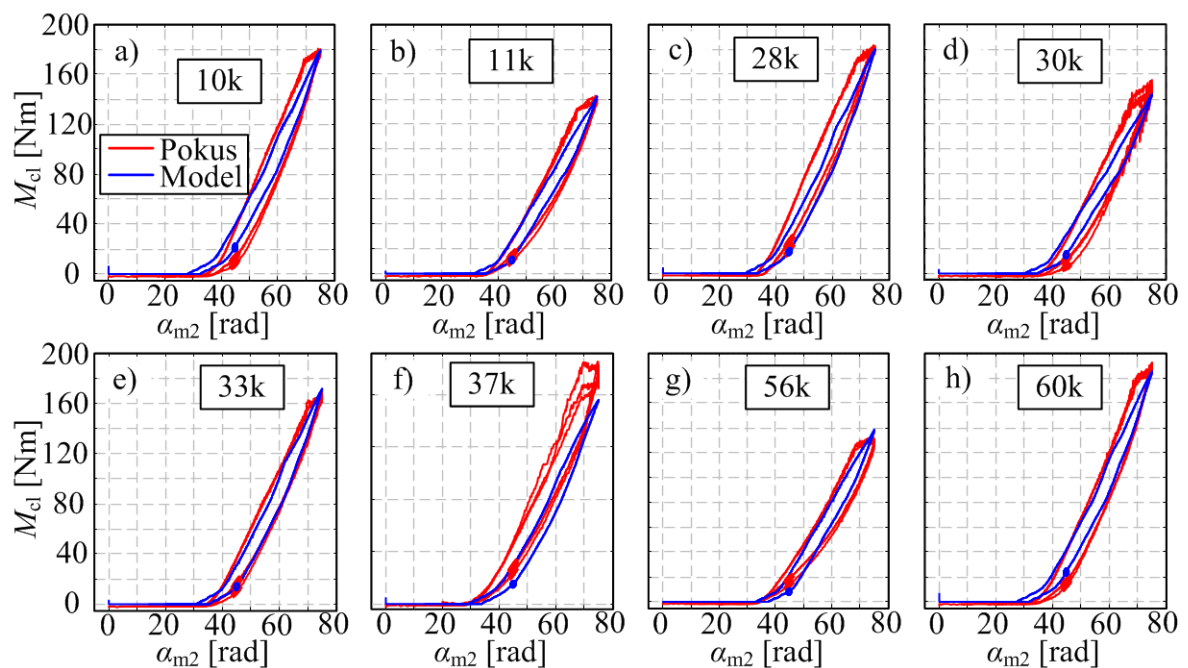
Slika 8-27: Filtrirane statičke karakteristike okretnog momenta trošenih spojki – najbolje poklapanje
