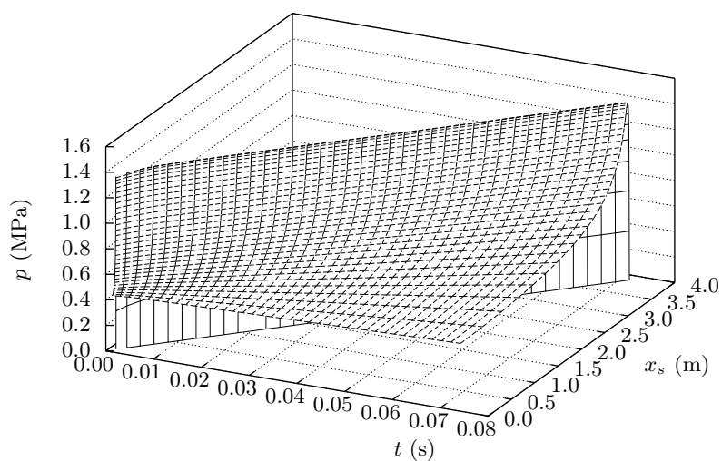
Slika 5.17: Prostorno-vremenska raspodijela tlaka (klin 15^\circ )
