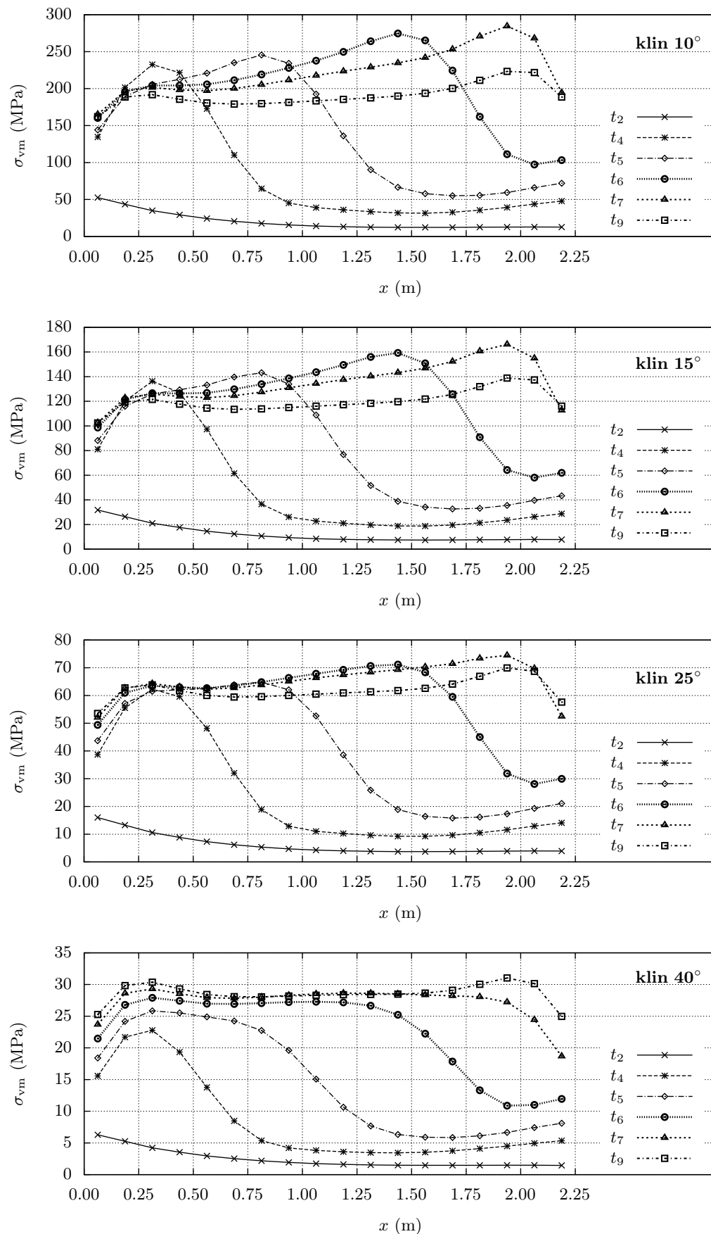
Slika 5.27: Promjena napreznja po teoriji von Misesa duž ukrepljenog panela, slika 5.25
