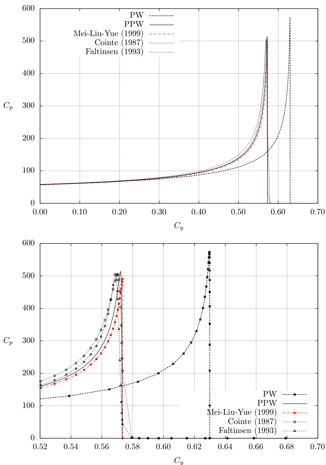
Slika 4.16: Usporedba prostorne raspodjele tlaka za klin nagiba 4^\circ
