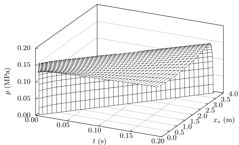
Slika 5.19: Prostorno-vremenska raspodijela tlaka (klin 40°)
