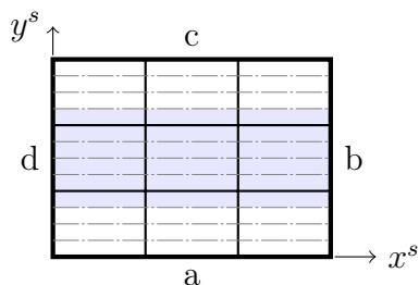
Slika 5.13: Skica modela s označenim stranicama i područjem djelovanja opterećenja
