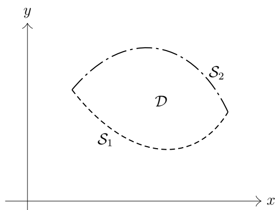
Slika B1: Skica domene općenitog Laplaceovog rubnog problema
