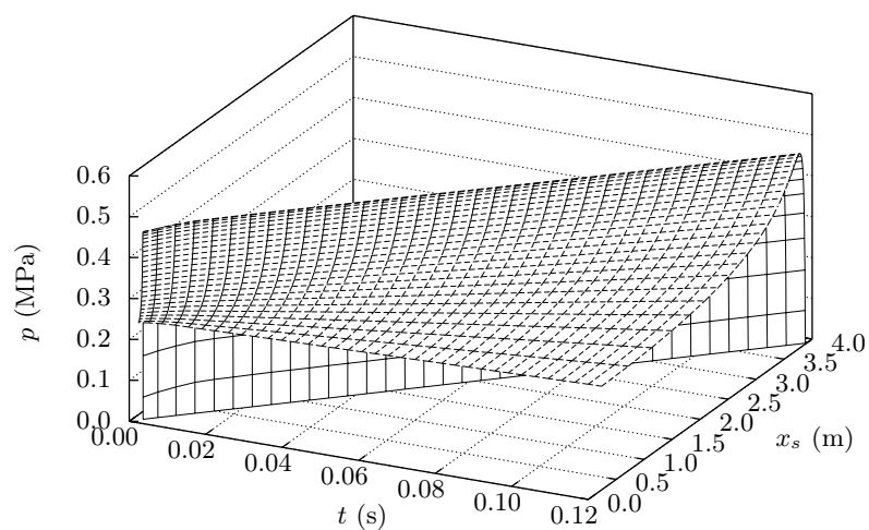
Slika 5.18: Prostorno-vremenska raspodijela tlaka (klin 25°)
