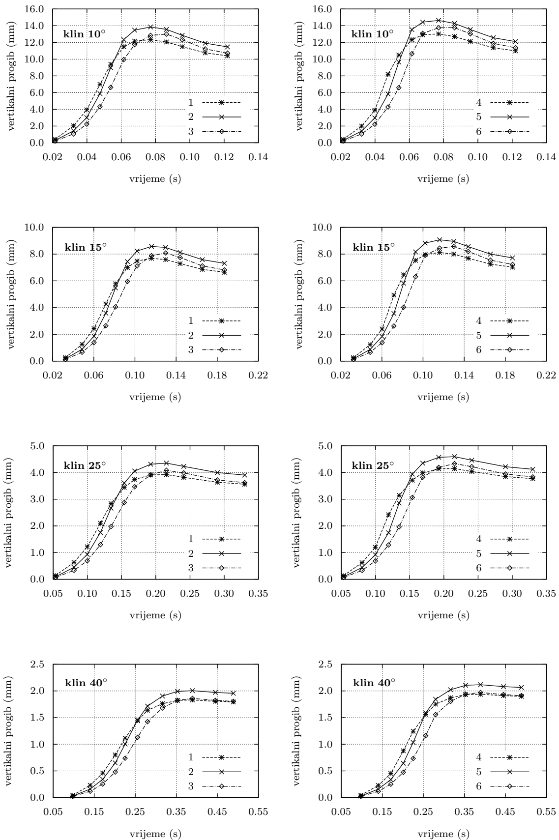
Slika 5.22: Vremenska promjena apsolutnih pomaka u smjeru z koordinata na odba- ranim pozicijama na modelu, slika 5.20
