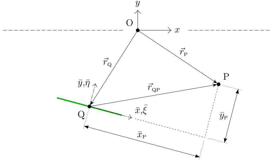
Slika 3.2: Parametrizacija segmenta i položaj točaka P i Q u proračunskom i segmentnom koordinatnom sustavu
