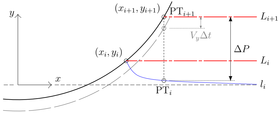
Slika 4.10: Određivanje vremenskog koraka pri simetričnom uronu
