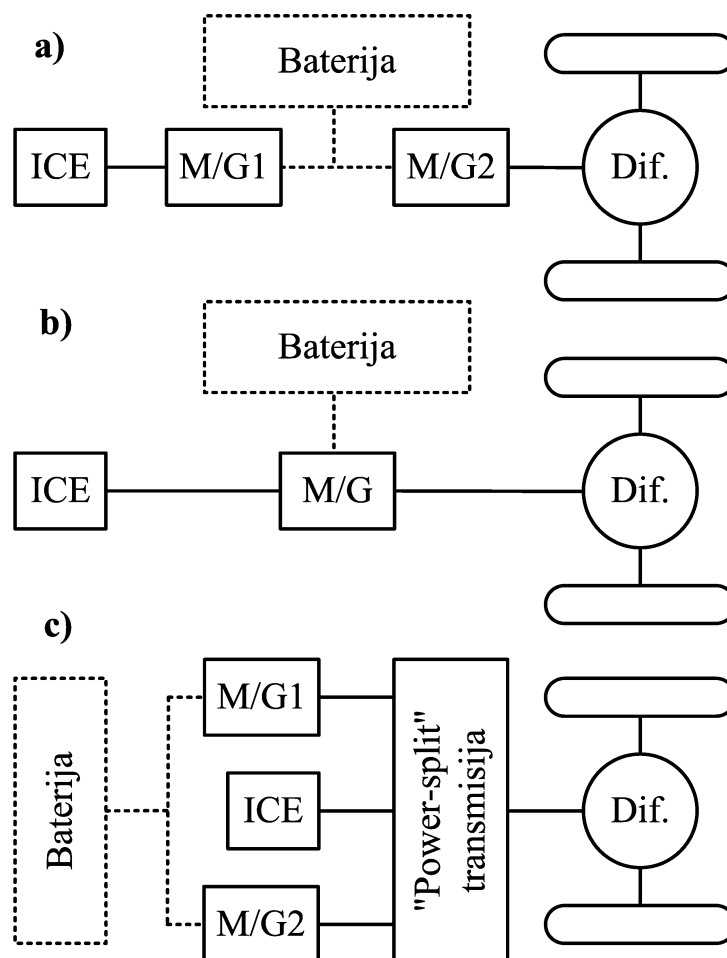
Slika 2-2: Temeljne konfiguracije hibridnog pogona: (a) serijska, (b) paralelna i (c) serijsko-paralelna.
