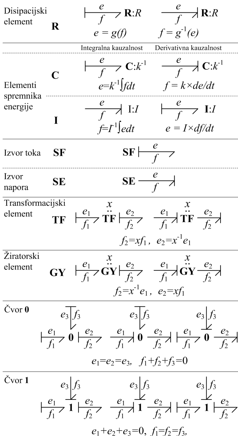
Slika 2-4: Osnovni elementi veznih dijagrama.
