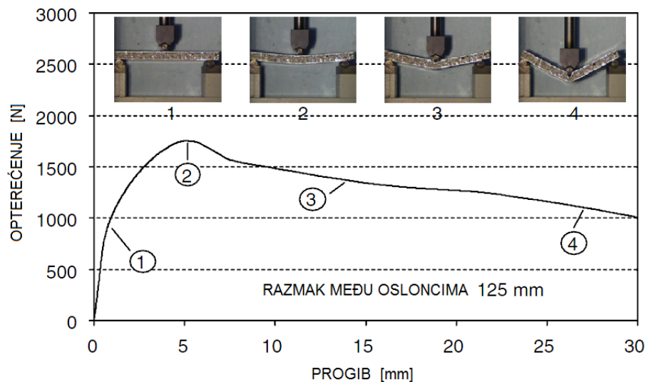
Slika 4.11. Dijagram opterećenje – progib pri ispitivanju aluminijskog sendvič panela savijanjem u tri točke s razmakom između oslonaca 125 mm [106]
