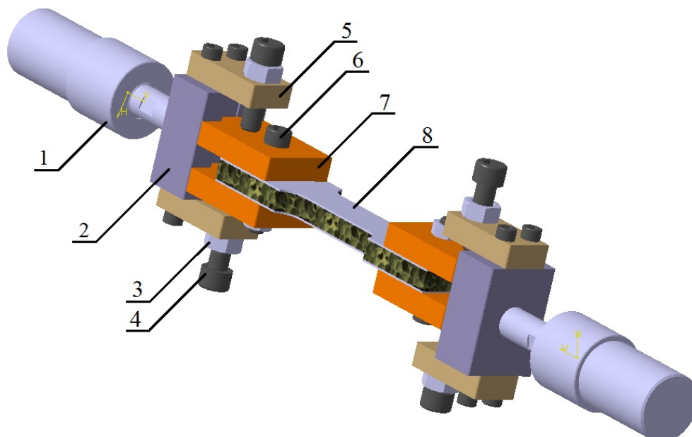
Slika 5.9. Skica stezne naprave za statičko vlačno ispitivanje:
