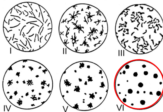
Slika 2.3 Klasifikacija grafita u Fe-C lijevovima sukladno HRN EN 945-1 (100:1) [32]
