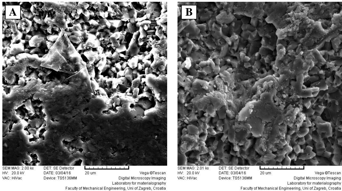
Slika 6.32 Morfologija površine monolitne \text{Al}_2\text{O}_3 keramike nakon erozijskog trošenja pri kutu upada od 90^\circ : (A) erodent: \text{SiO}_2 ; (B) erodent: \text{SiC} (povećanje \sim 2000 \times )
