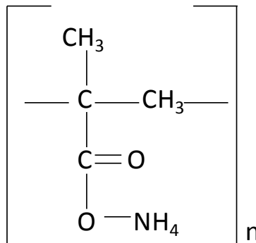
Slika 5.1 Sirovine korištene za pripremu uzoraka monolitne Al_2O_3 i kompozitne Al_2O_3-ZrO_2 keramike (disperezant i dvije vrste keramičkog praha)
