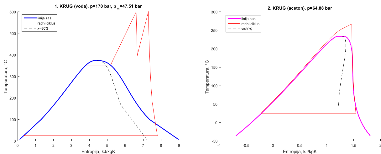
Slika 8.5 T - s dijagram postrojenje s acetonom kao radnim medijem u drugom krugu pare, \Delta T_{pp} = 10 \text{ }^\circ\text{C} i T_{dp,ul} = 627 \text{ }^\circ\text{C} – termodinamička optimizacija postrojenja s dva kruga pare i međupregrijanjem
