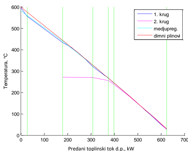
Slika 7.48 T-\Phi dijagram postrojenje s R11 kao radnim medijem u drugom krugu pare i T_{dp,ul} = 600\text{ }^{\circ}\text{C} – termodinamička optimizacija postrojenja s dva kruga pare i međupregrijanjem
