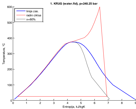
Slika 11.20 Rezultati termodinamičke optimizacije pojrojenja s dva kruga pare, T_{dp,ul} = 600 °C, R123 kao radni medij drugog kruga pare
