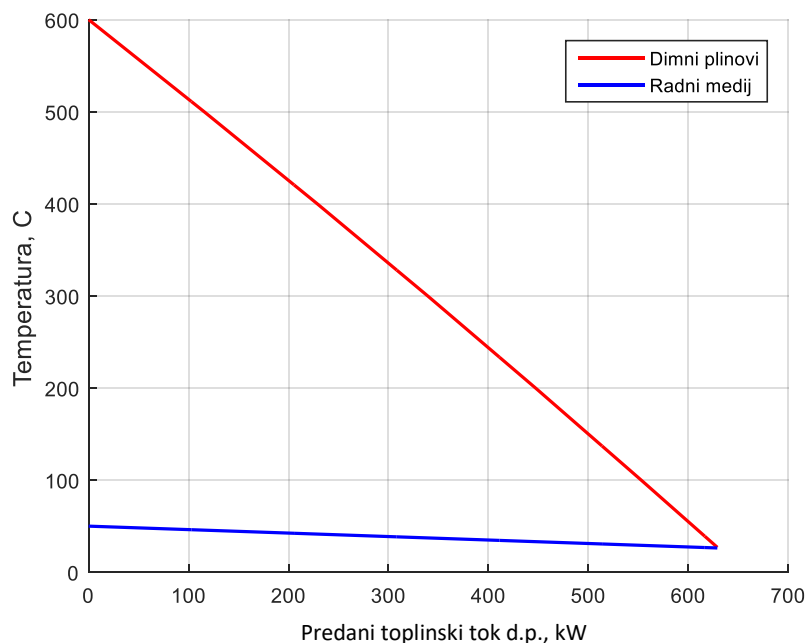
Slika 5.2. Predani toplinski tok dimnih plinova radnom mediju velikog toplinskog kapaciteta
