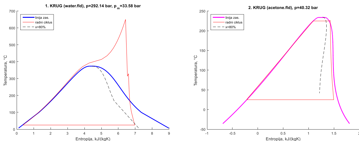
Slika 7.80 T-s dijagram postrojenja s acetonom kao radnim medijem u drugom krugu pare i T_{dp,ul} = 700\text{ }^{\circ}\text{C} – eksergoekonomska optimizacija postrojenja s dva kruga pare i međupregrijanjem
