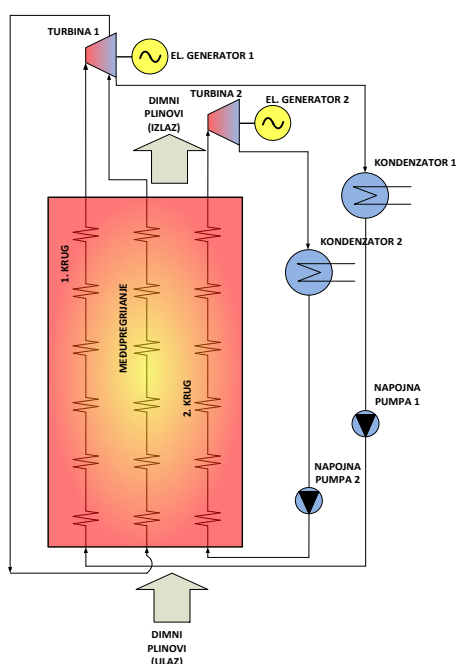
Slika 7.39 Shema parnoturbinskog postrojenja s dva kruga pare i međupregrijanjem
