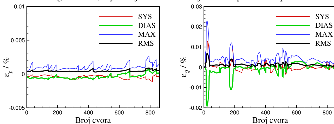
Slika 23. Relativne pogreške (u postocima) modela rješavanog razvijenom metodom karakteristika (s lineariziranim matematičkim modelom) u odnosu na metodu transmisijске linije. Lijevi dijagram pokazuje pogreške u tlaku: \epsilon_p^{\text{RMS}} , \epsilon_p^{\text{SYS}} , \epsilon_p^{\text{DIAS}} i \epsilon_p^{\text{MAX}} . Desni dijagram pokazuje pogreške u protoku: \epsilon_Q^{\text{RMS}} , \epsilon_Q^{\text{SYS}} , \epsilon_Q^{\text{DIAS}} i \epsilon_Q^{\text{MAX}} . Pogreške su definirane jednadžbama (42) - (49).
