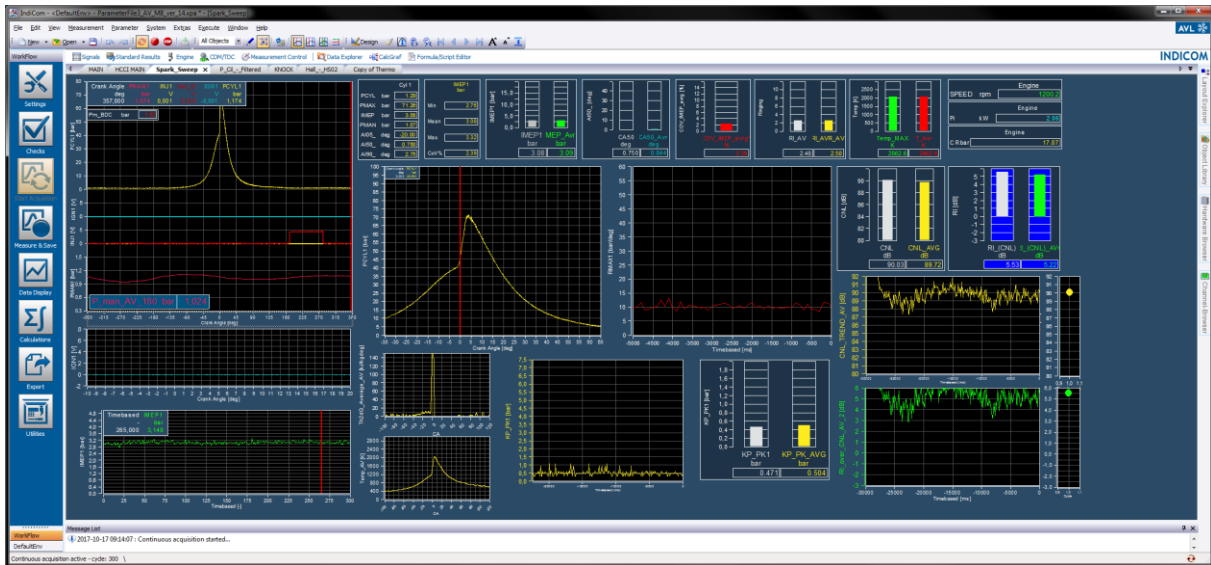
Slika 2.54. Izgled sučelja za indiciranje i nadziranje rada motora u programskom paketu AVL IndiCom [10]
