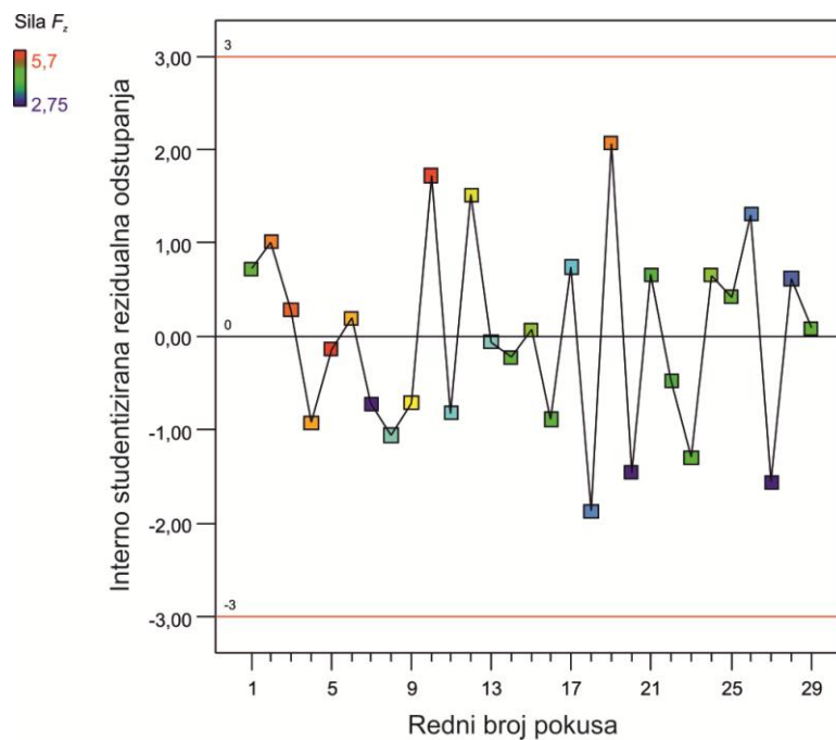
Slika 5.9 Slučajno rasipanje rezidualnih odstupanja u odnosu na redosljed izvođenja plana pokusa za linearni matematički model za izračunavanje aksijalne sile mikrobušenja
