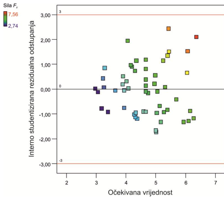
Slika 5.20 Dijagram rezidualnih odstupanja u ovisnosti o očekivanim vrijednostima modela za izračunavanje aksijalne sile mikrobušenja potpomognutoga vibracijama
