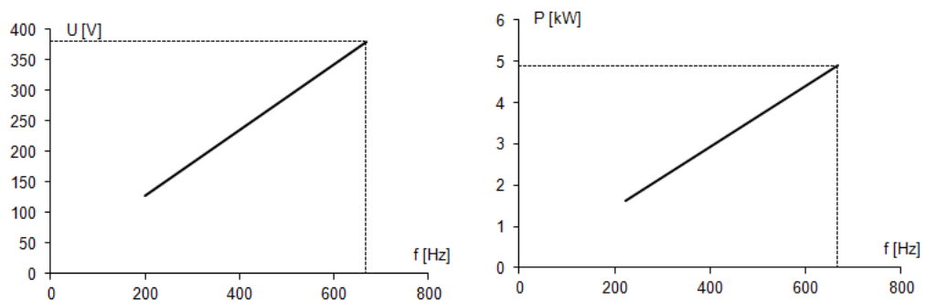
Slika 4.4 Pogonske karakteristike ugradbenog motora E+A mW 7/7-2-267d/282dr0
