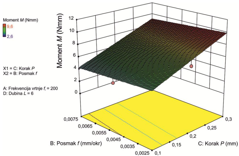
Slika 5.18 3D prikaz matematičkog modela ovisnosti momenta M mikrobušenja o posmaku f i dubini koraka P (dubina provrta L = 6 mm, n = 12\ 000 min -1 )
