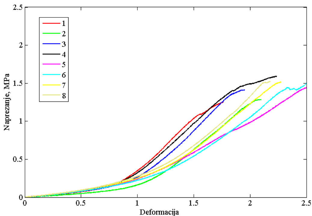
Slika 76. Dijagram deformacija-naprežanje svježih poprečnih uzoraka aorte za pohranu od mjesec dana
