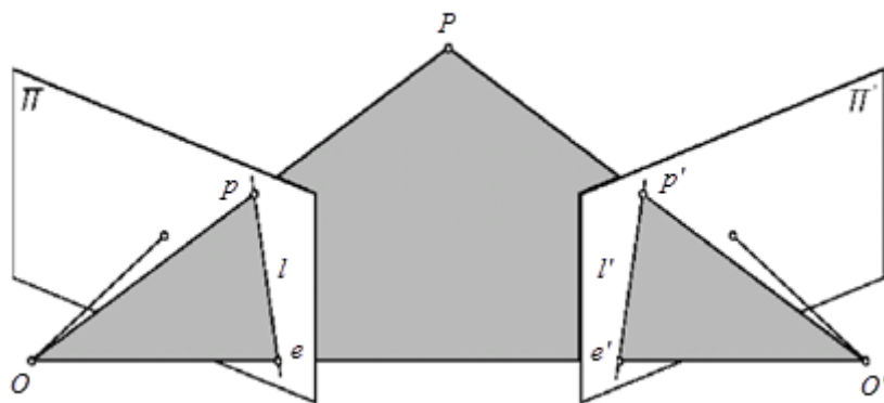
Slika 32. Epipolarna ravnina [160]
