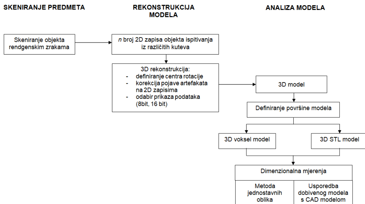
Slika 2-2. Proces provedbe dimenzionalnog mjerenja računalnom tomografijom.
