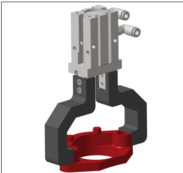
Slika 21. Hvataljka za odstojnik mehanizma
