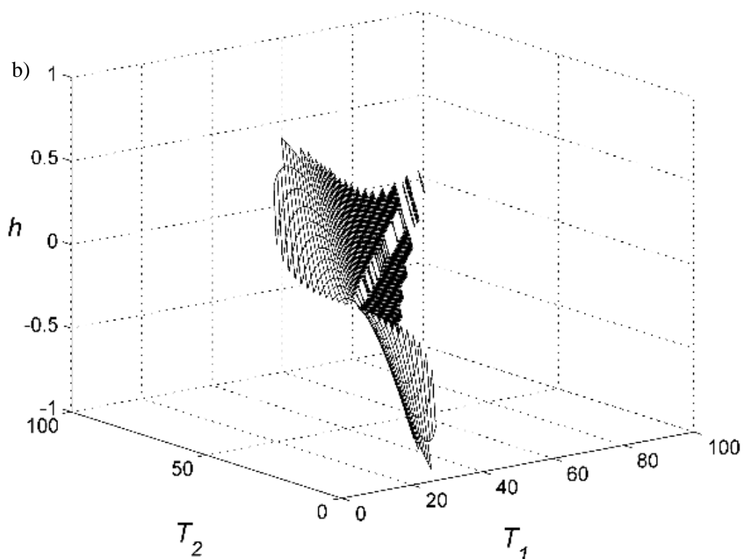
Slika 66. Geometrijske udaljenosti između letjelica u ovisnosti o T_1 i T_2 a) d/L ; b) h/L pri \psi = \pi/2 i m_{1,2}/m_0 = 1 .
