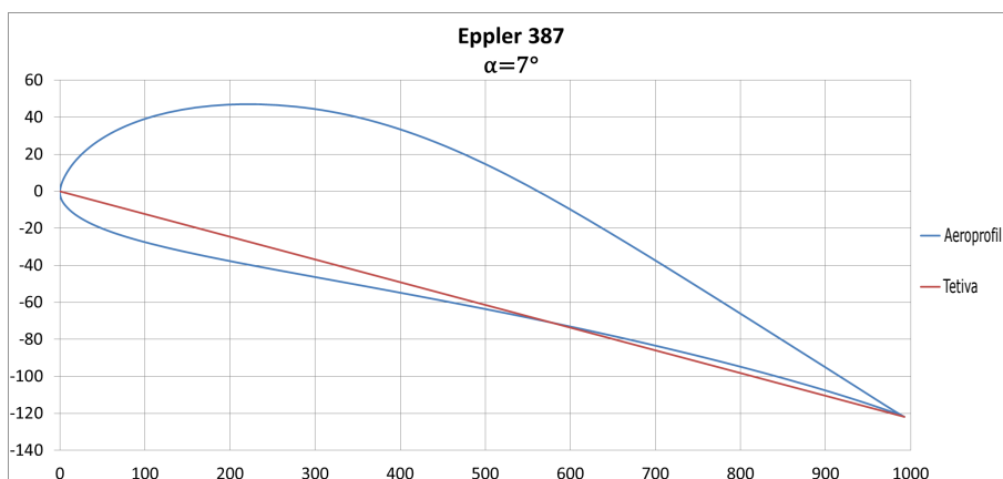
Slika 3: Aeroprofil Eppler 387 pri napadnom kutu \alpha = 7^\circ .
