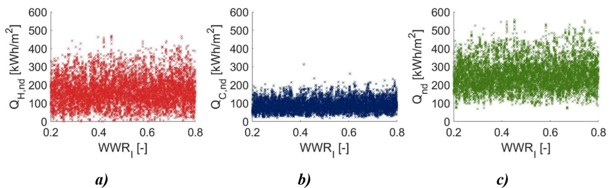
Slika 36. Ovisnost potrebne energije za a) grijanje, b) hlađenje, c) grijanje i hlađenje o promjeni vrijednosti udjela površine prozora na istočnoj fasadi
