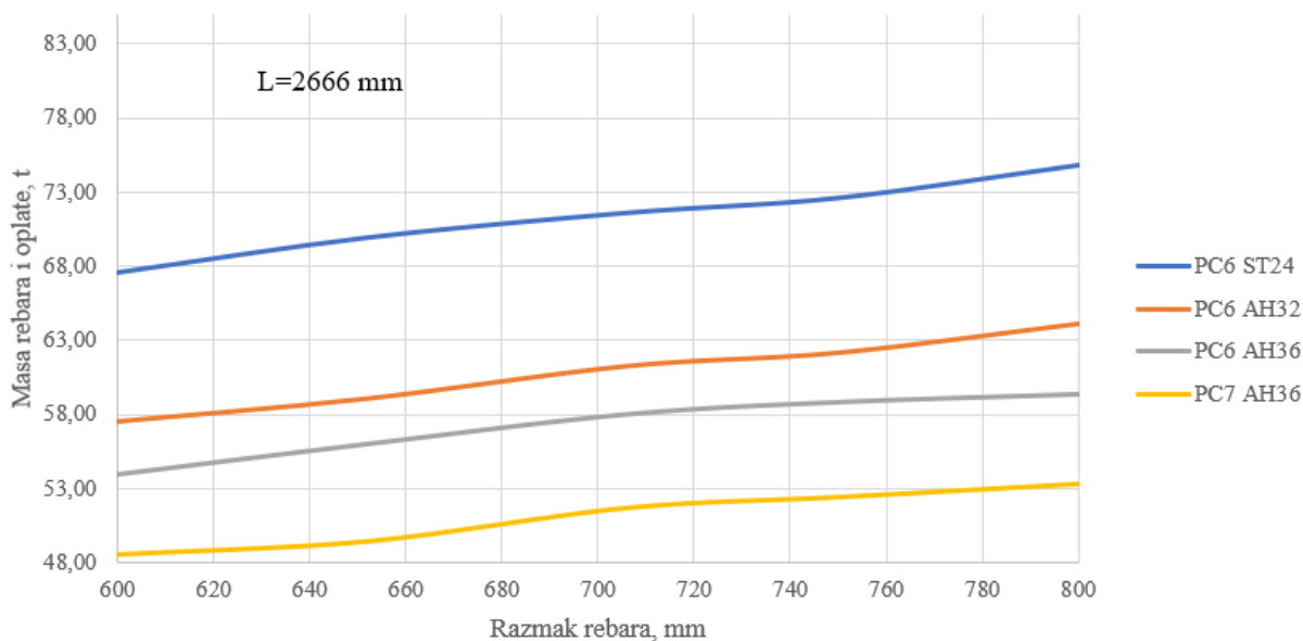
Slika 11. Ovisnost mase rebara i oplata o razmaku rebara za čelik različite kvalitete, dvije proveze jednoliko razmahnute
