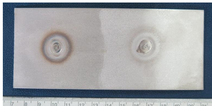
Slika 31. Uzorak čelika AISI 904L (EN 1.4539) nakon korozijskog ispitivanja, vidljivo je da nema oštećenja te da se materijal može smatrati postojanim na rupičastu koroziju
