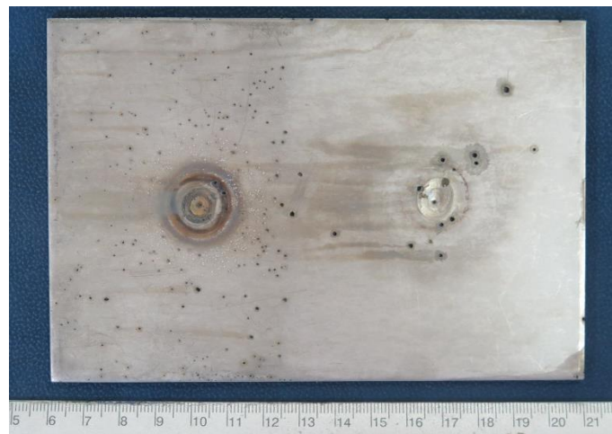
Slika 30. Uzorak čelika AISI 316Ti (EN 1.4571) nakon korozijskog ispitivanja. Nešto manja otpornost od čelika AISI 316L.
