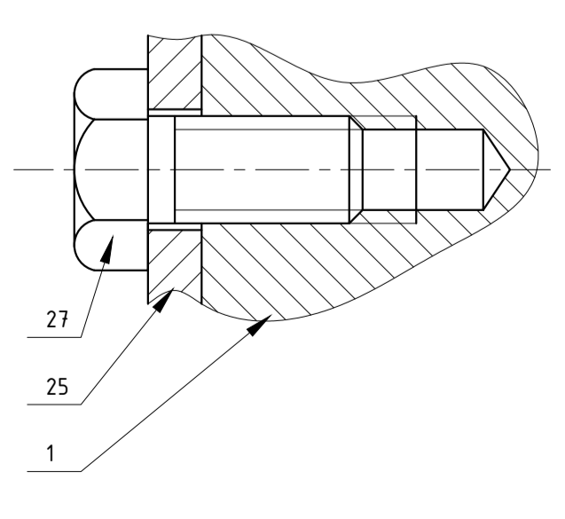
Presjek D-D (M 2:1) Prikaz spoja poklopca ležaja
