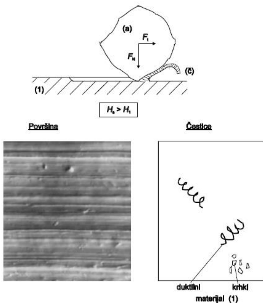
Slika 14. "Čista" abrazija [9]
