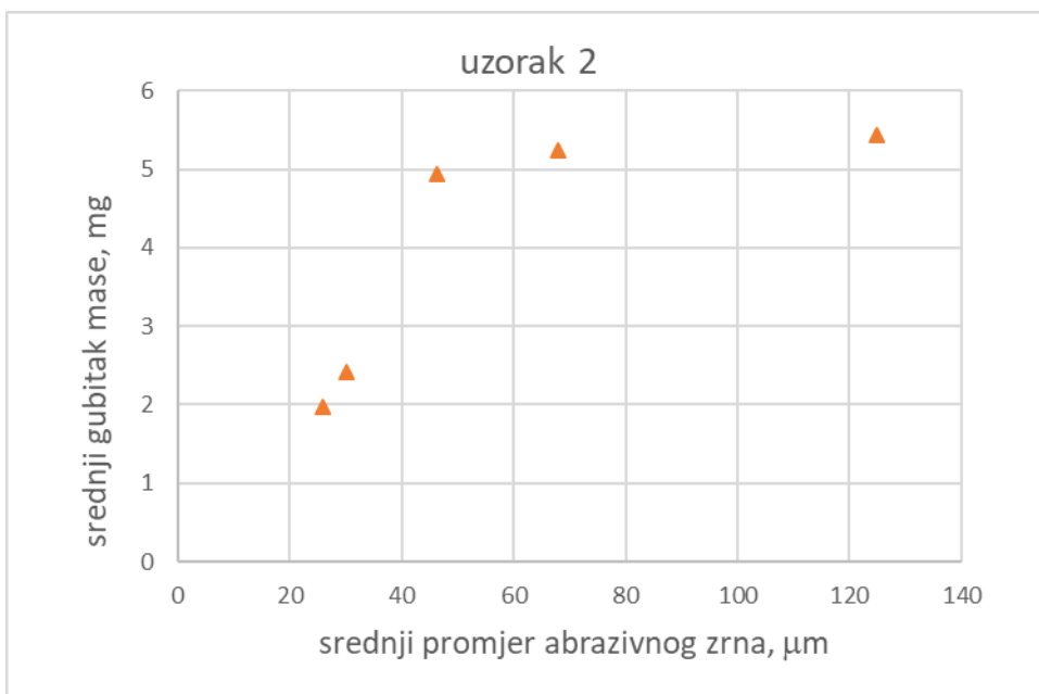
Slika 49. Ovisnost abrazivskog trošenja o veličini abrazivnog zrna za uzorak 2
