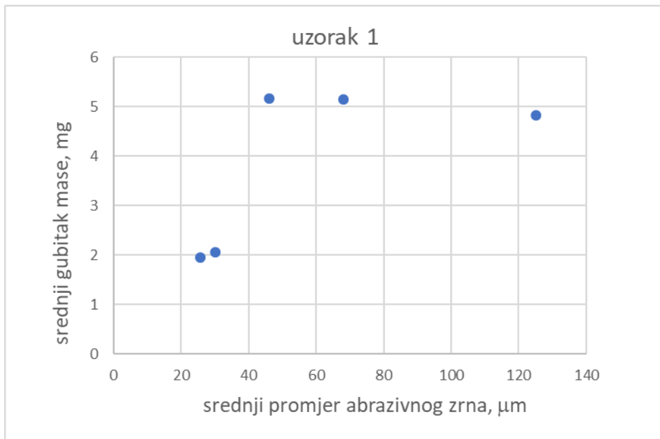
Slika 48. Ovisnost abrazivskog trošenja o veličini abrazivnog zrna za uzorak 1
