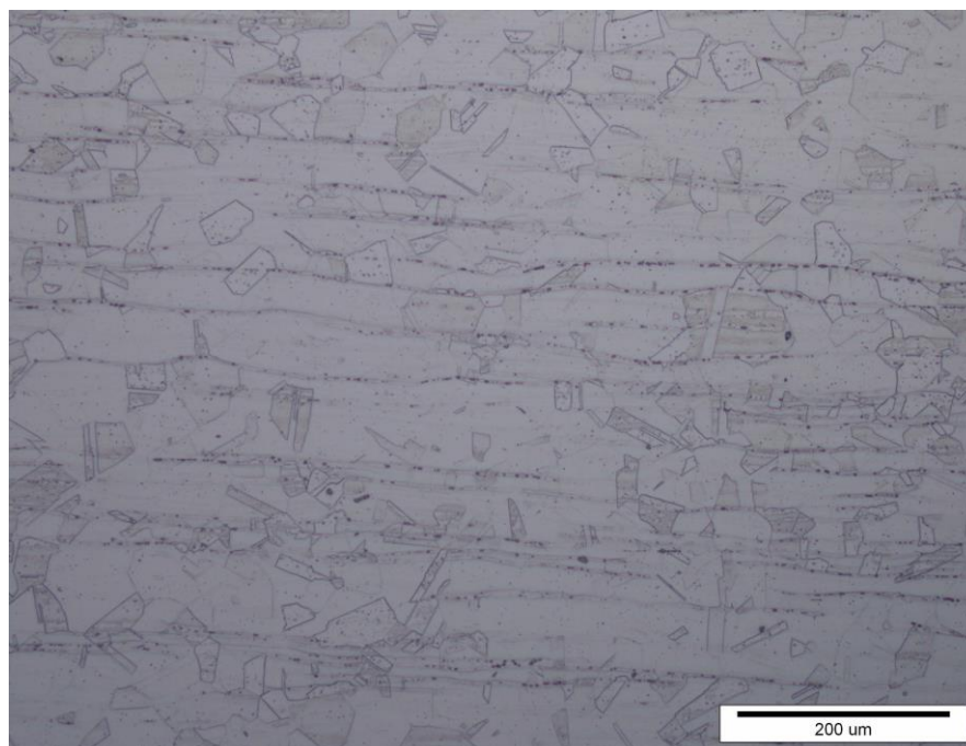
Slika 34. Mikrostruktura uzorka 1 snimljena pri povećanju 200×
