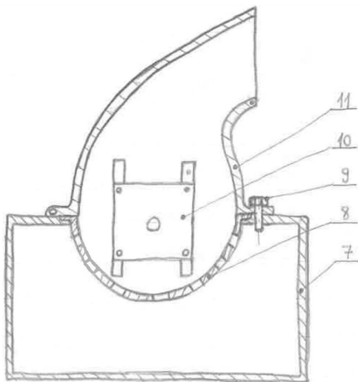
Slika 21. Presjek kućišta
