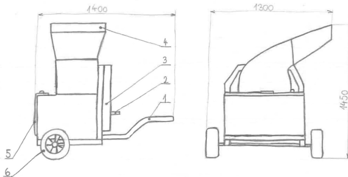
Slika 20. Koncept 3
