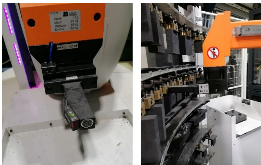
Slika 24. Automatski čitač ID-koda
