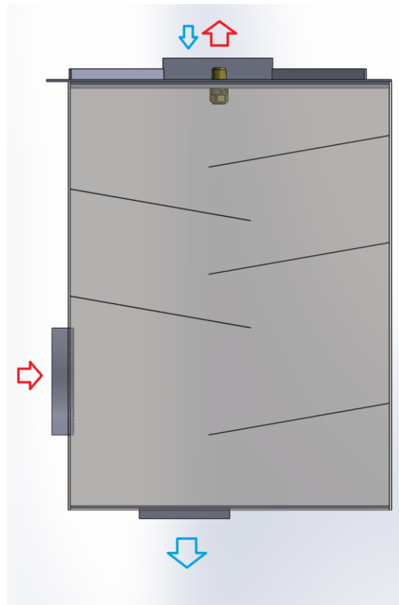
Slika 16. Presjek prostora za filtraciju.
