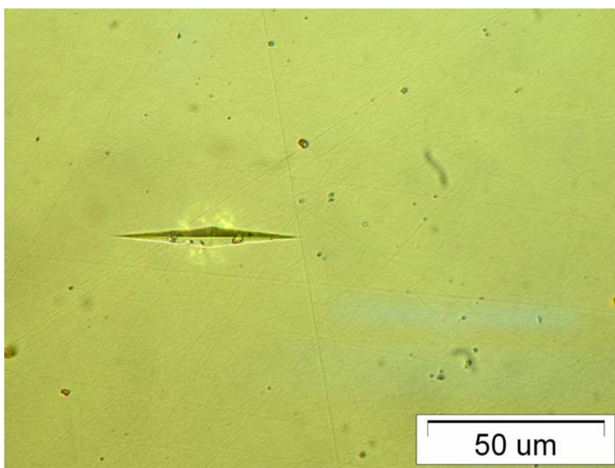
Slika 36 Otisak dijamantne piramide nakon mjerenja tvrdoće metodom HK0,5
