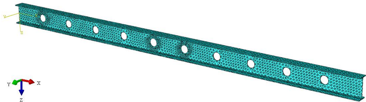
Slika 41. Diskretizirani numerički model s 28316 C3D10 konačnih elemenata za D/h = 0,4
