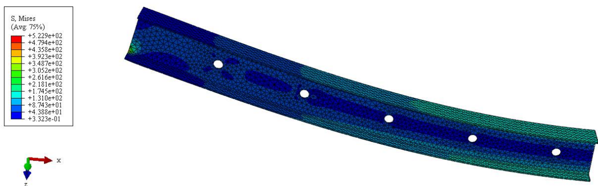
Slika 42. Raspodjela ekvivalentnih naprezanja prema von Misesu za D/h = 0,2 u MPa
