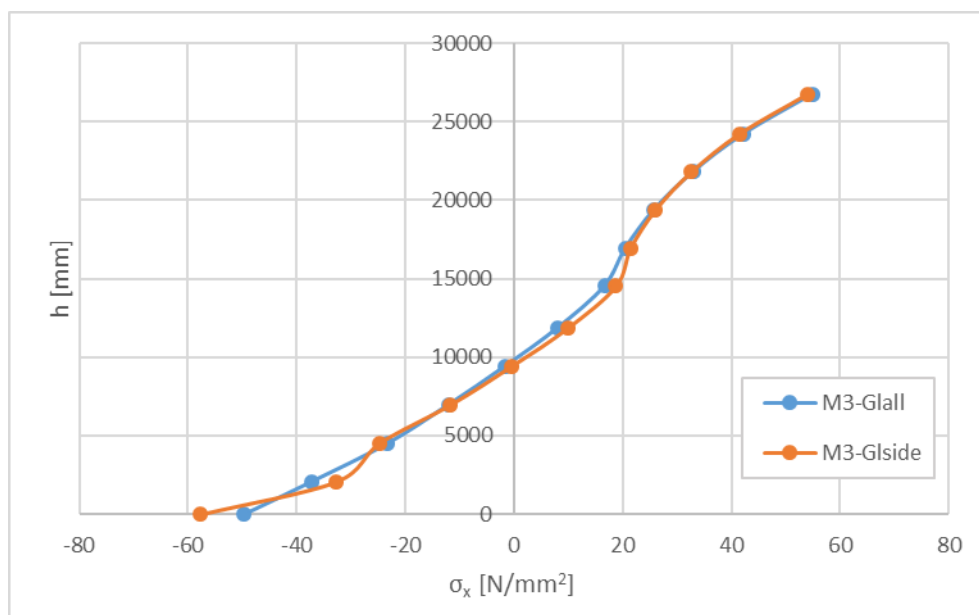
Slika 19 Raspodjela \sigma_x naprezanja po visini M3 modela na glavnom rebu, na poziciji CL
