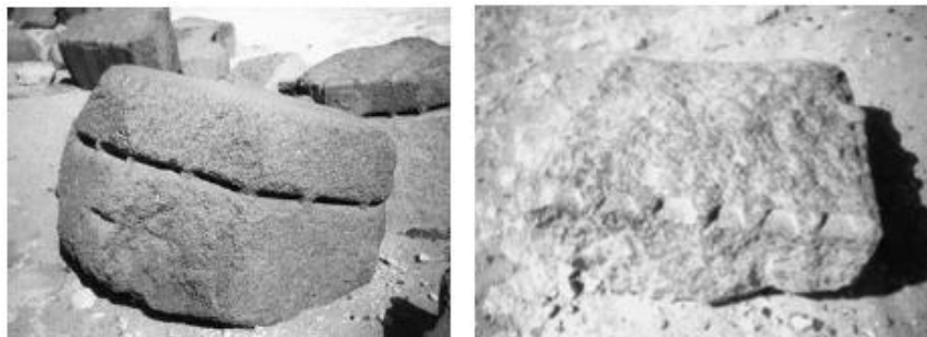
Slika 3.4. Cijepanje granitnog kamena uz pomoć tlaka bubrenja [4]
