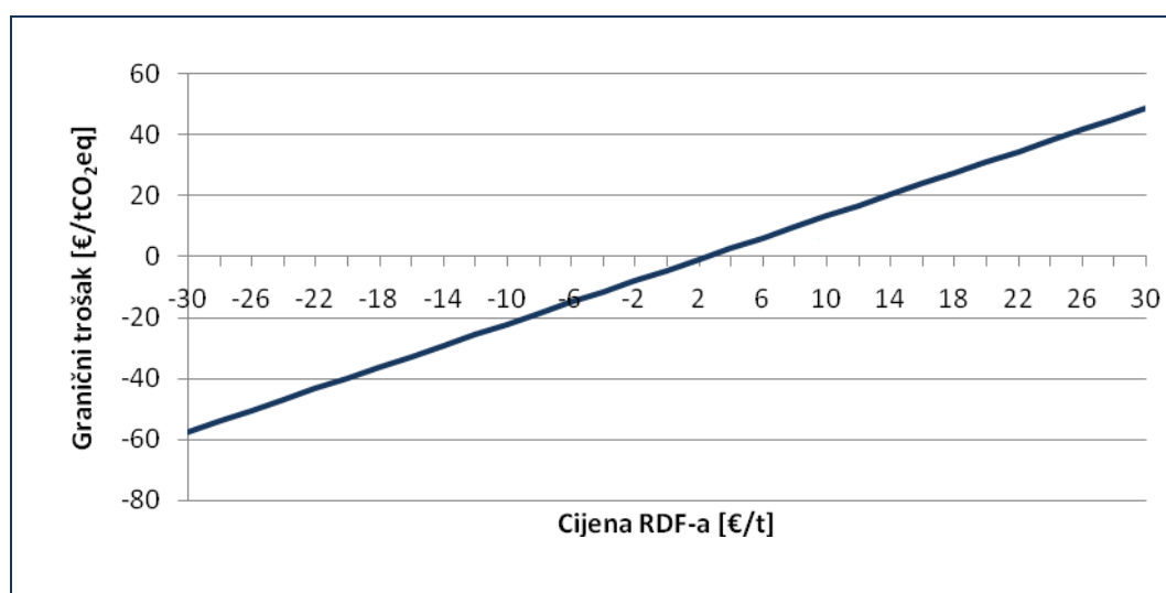
Slika 17. Ovisnost graničnog troška korištenja RDF-a u cementnoj industriji o cijeni RDF-a
