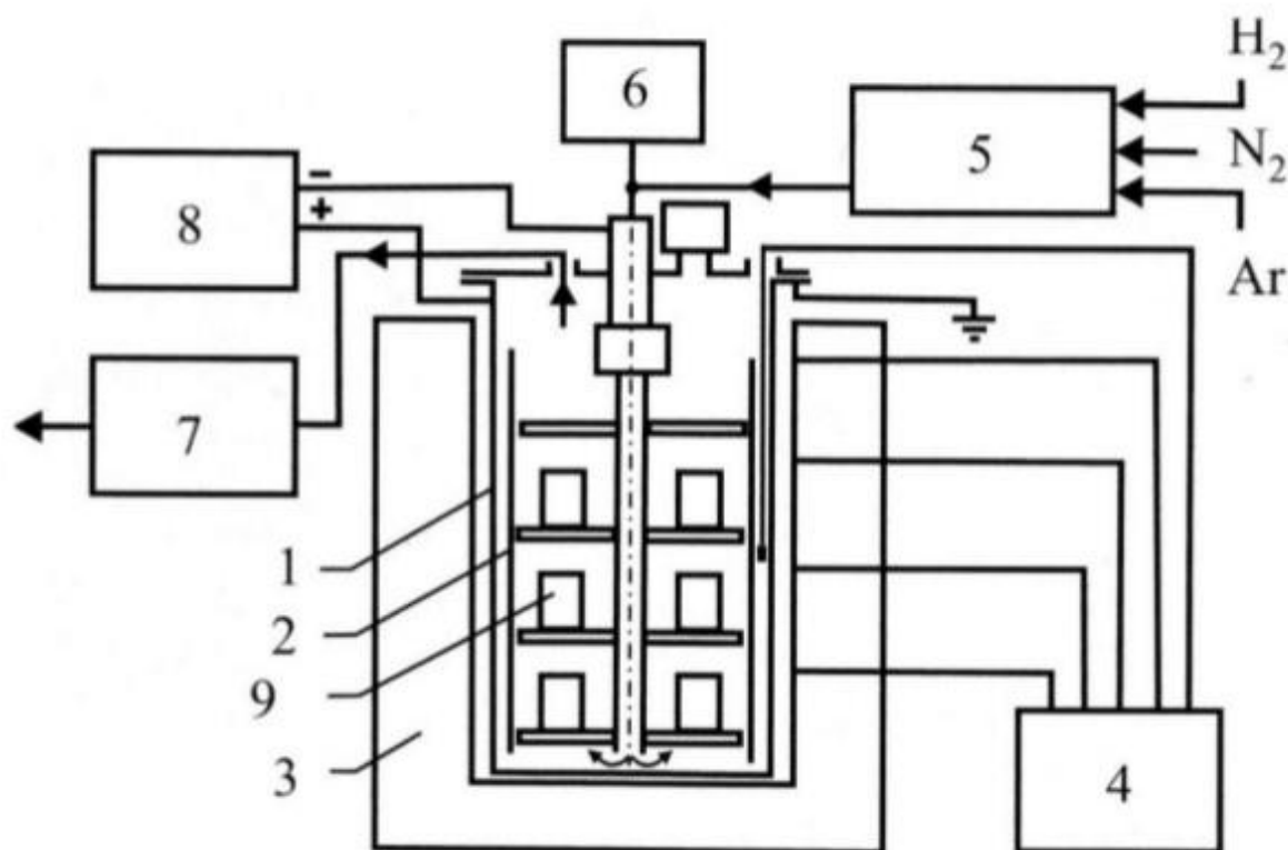
Slika 4.6. Shematski prikaz opreme za PACVD postupak [10]
