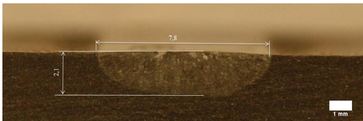
Slika 34. Grafički prikaz penetracije navara pojedinih makrouzoraka
