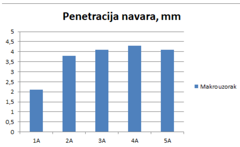
Slika 34. Grafički prikaz penetracije navara pojedinih makrouzoraka
