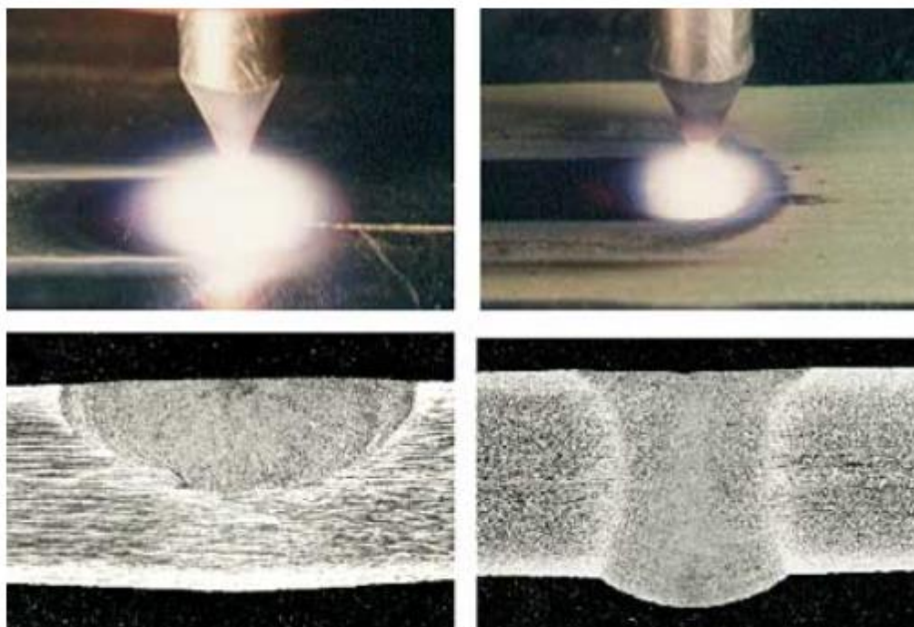
Slika 7. Karakteristični izgled luka kod A-TIG i konvencionalnog TIG zavarivanja i usporedba dubine penetracije kod nehrđajućeg čelika debljine 6 mm (desno: konvencionalni TIG, lijevo: A-TIG [16])
