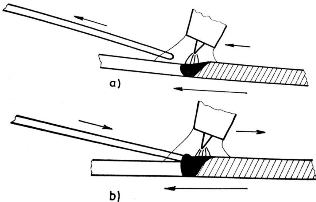
Slika 6. Prikaz tehnike rada u dodavanju žice u talinu kod ručnog TIG zavarivanja[2]: a) od kretanja pištolja naprijed izmaknuti žicu, pretaliti osnovni materijal b) povući pištolj malo unazad, a žicu dodati u rub taline itd; proces se nastavlja
