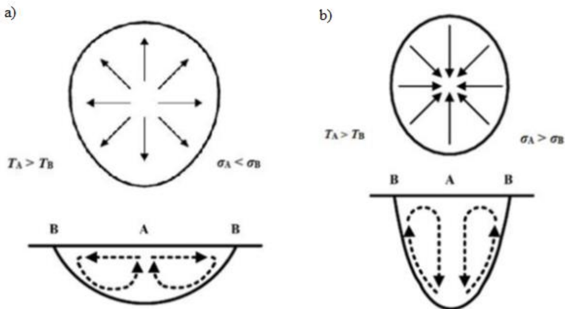
Slika 10. Marangonijev efekt strujanja fluida [8]: a) Centrifugalni b) Centripetalni
