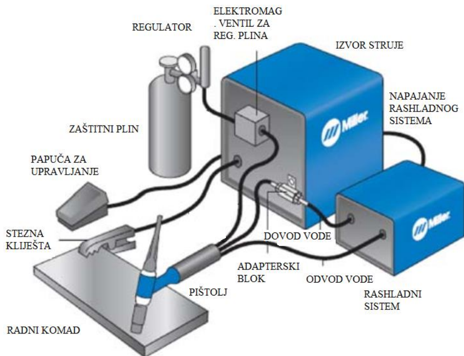
Slika 2. Dijelovi uređaja za TIG zavarivanje [5]
