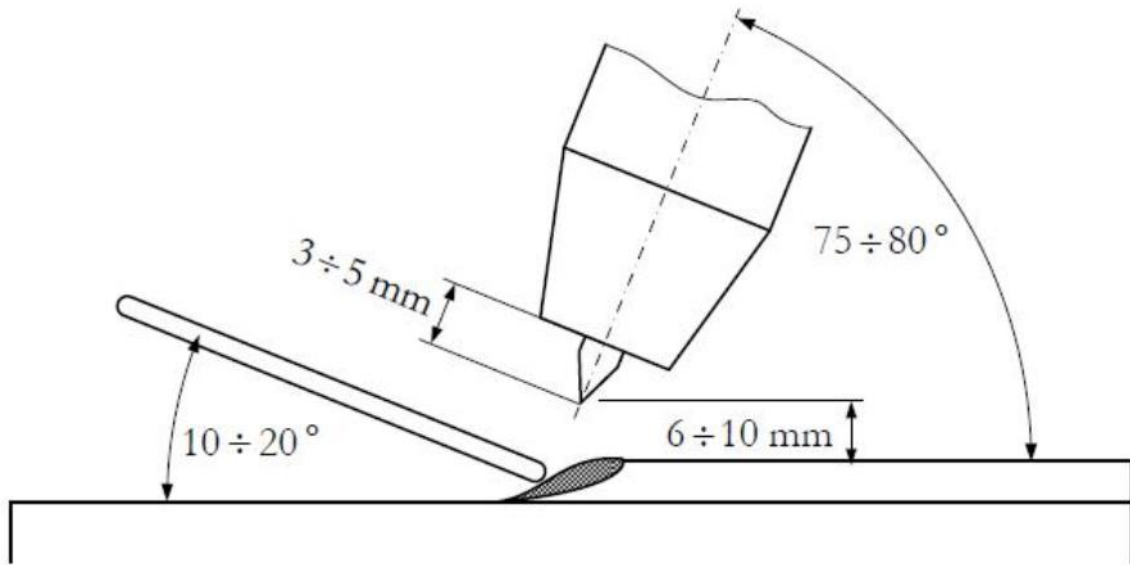
Slika 5. Položaj elektrode i dodatnog materijala u odnosu na radni komad [7]
