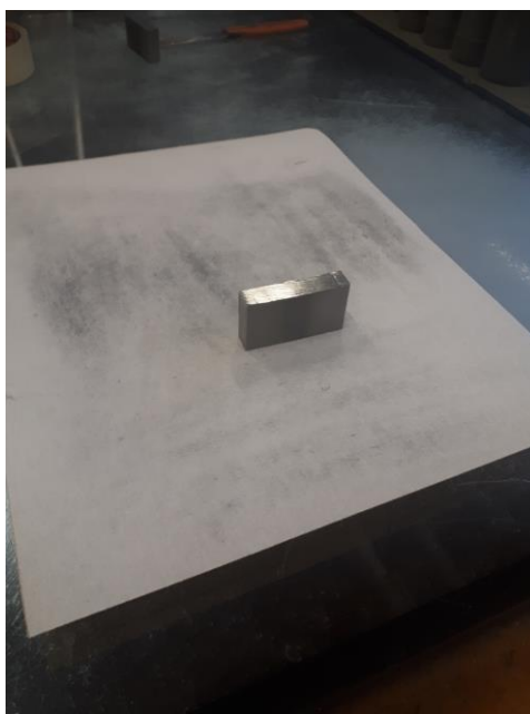
Slika 26. Brušenje uzorka na brusnom papiru P150
