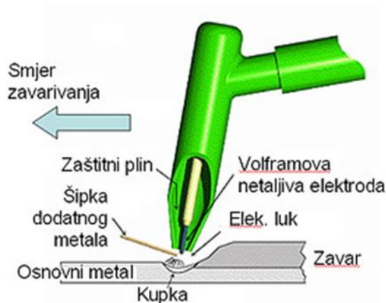
Slika 1. Shematski prikaz TIG postupka zavarivanja [4]
