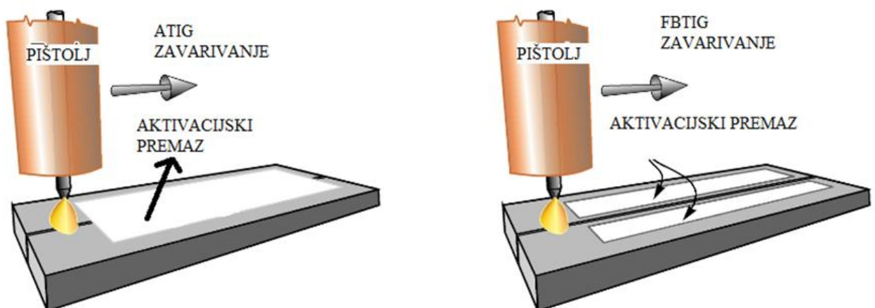
Slika 9. Shema ATIG i FBTIG zavarivanja [12]
