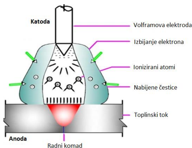
Slika 11. Mehanizam kontrakcije električnog luka [14]
