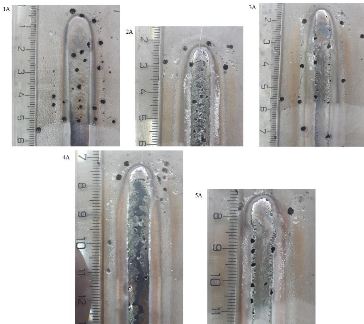
Slika 41. Izgled navarenih uzoraka nakon 48-satnog izlaganja agresivnoj otopini
