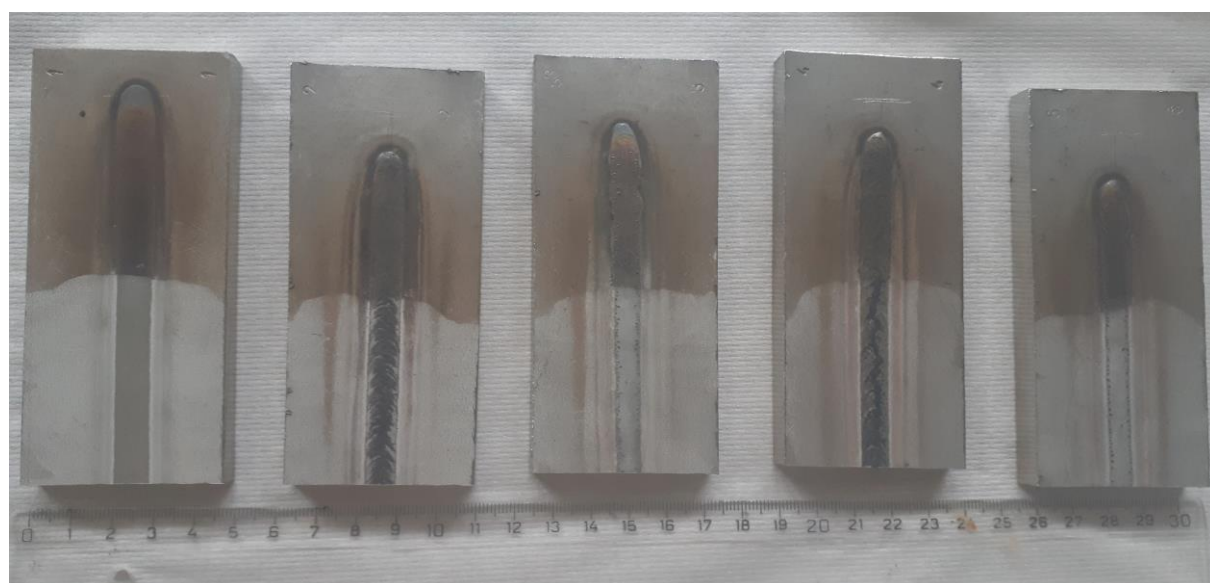
Slika 32. Uzorci nakon djelovanja paste
