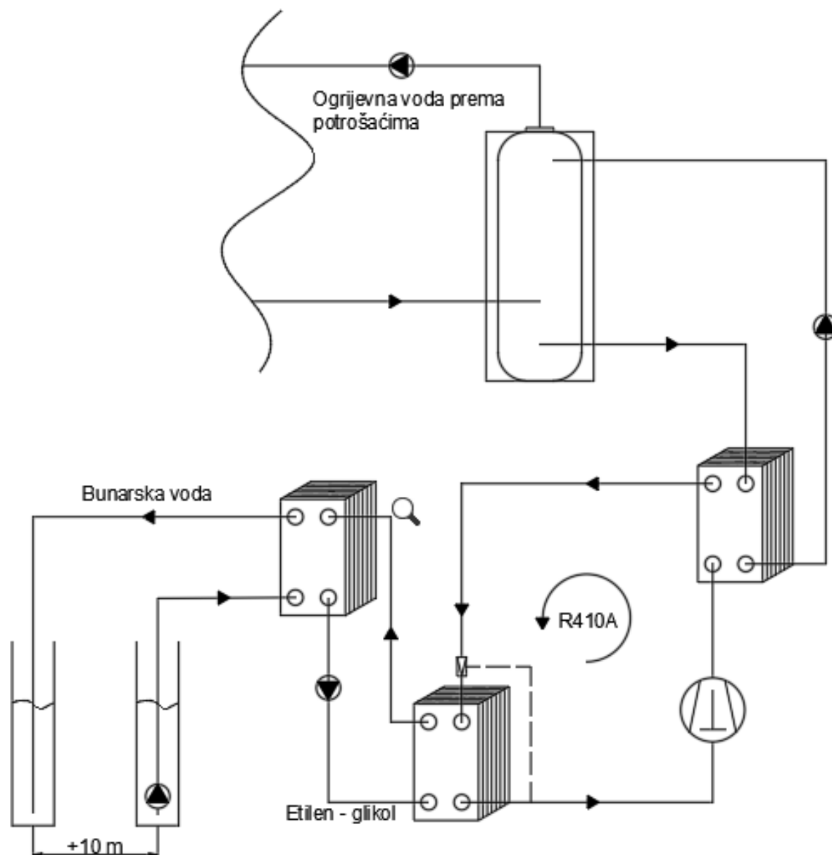
Slika 18. Shematski prikaz sustava grijanja s dizalicom topline
