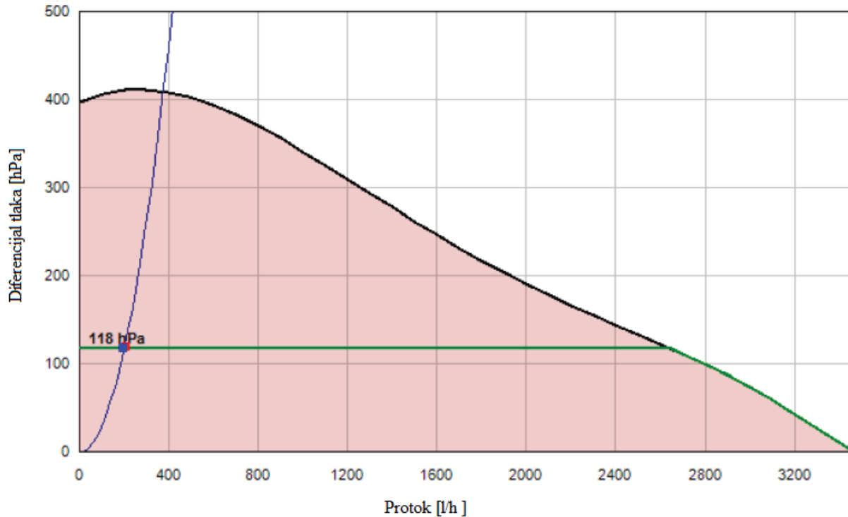
Slika 30. Krivulja crpke
