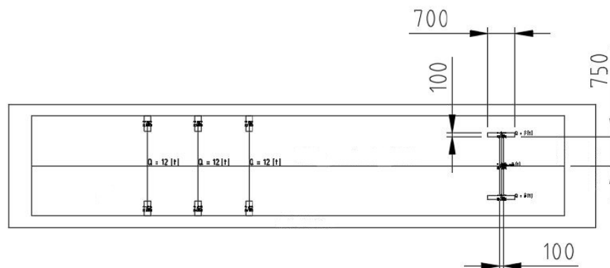
Slika 11. Raspored i dimenzije dodirne površine stalka
