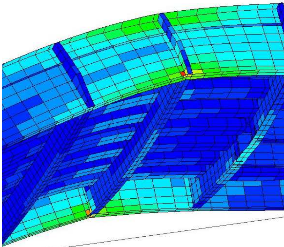
Slika 29. Najveća von Mises naprežanja LCH-2
