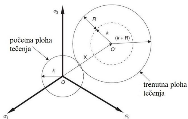
Slika 8. Ploha tečenja mještovitog izotropnog – kinematičkog očvršćenja [10]
