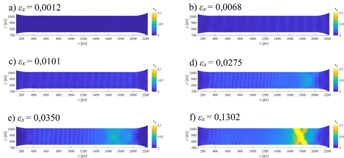
Slika 23. Raspodjela deformacija po mjerenom području za slučaj cikličkog ispitivanja
