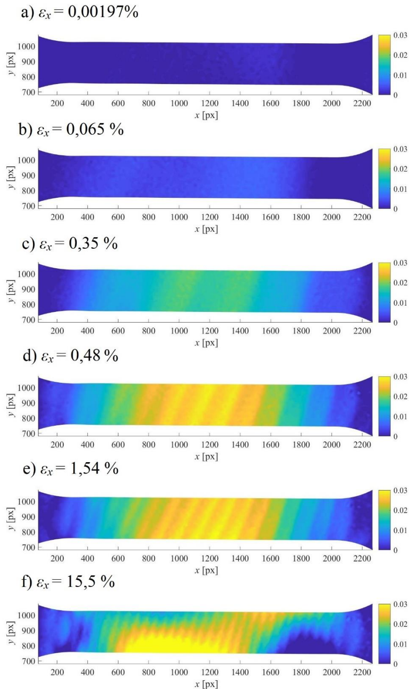
Slika 37. Razlika izmjenenog i izračunatog polja pomaka kod identifikacije parametara kinematičkog očvršćenja kod jednoosnog monotonog opterećenja prikazane za vrijednosti prosječne deformacije na cijelom mjernom području: a) 0,00197 %, b) 0,065 %, c) 0,35 %, d) 0,48 %, e) 1,54 % i f) 15,5 %
