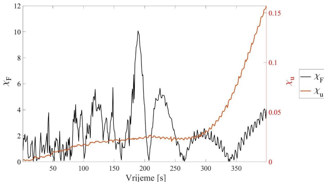
Slika 31. Razlika funkcionala \chi_F i \chi_u u zadnjoj iteraciji identifikacije parametara izotropnog očvršćenja kod jednoosnog monotono opterećenja
