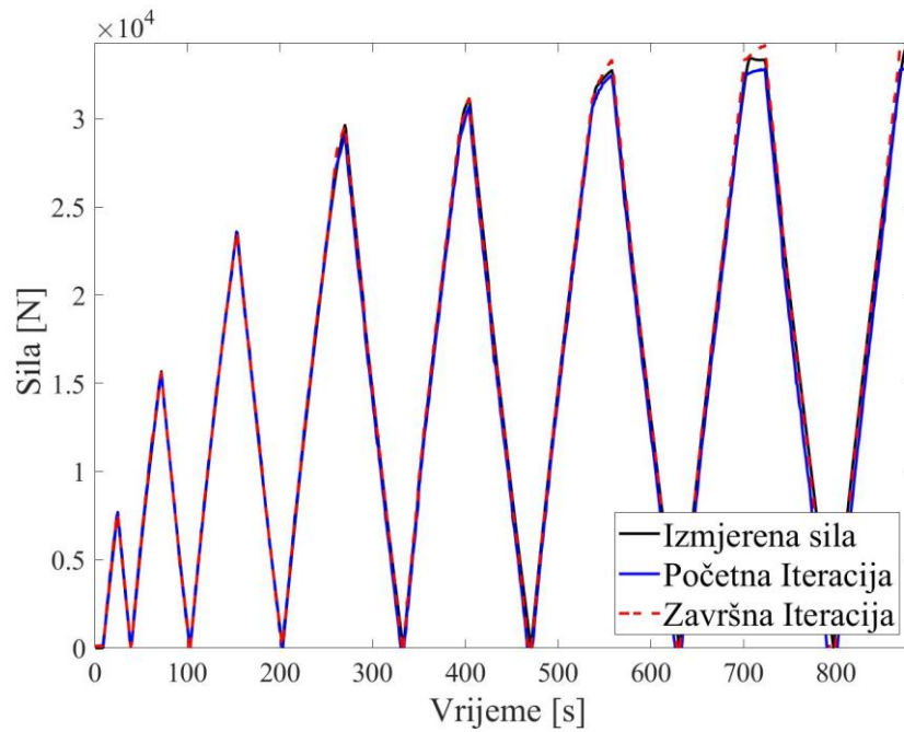
Slika 48. Usporedba izmjerene sile i sume reaktivnih sile izračunatih u prvoj i zadnjoj iteraciji za slučaj identifikacije parametara izotropnog očvršćenja kod jednoosnog cikličkog ispitivanja
