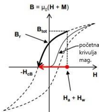
Slika 13. Djelovanje suprotnog magnetskog polja na početno magnetsko polje radnog komada [9]
