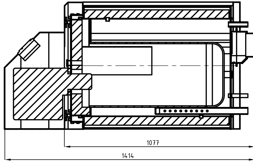
PRESJEK A-A
