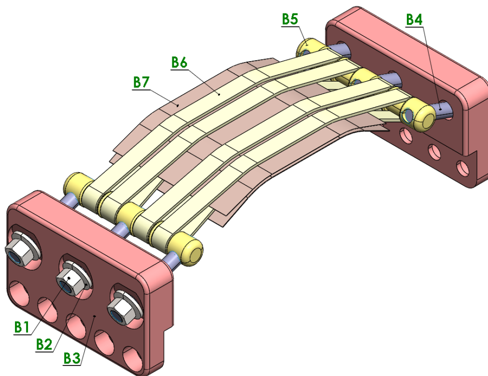
Slika 35. Princip stezanja Polyglas® trakama
