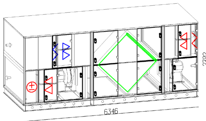
Slika 5.3 Centralna klima komora etaže 1. kata
