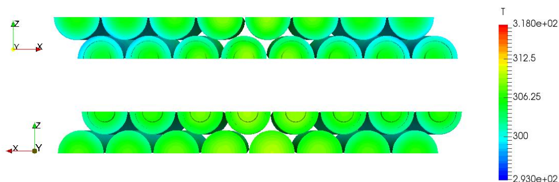
Slika 5.7 Temperaturno polje [K] ćelija pri brzini strujanja na ulazu od 40 m/s i uniformnim razmakom između ćelija –strana ćelija bliže ulazima (gornja slika) i strana ćelija bliže izlazima (donja slika)
