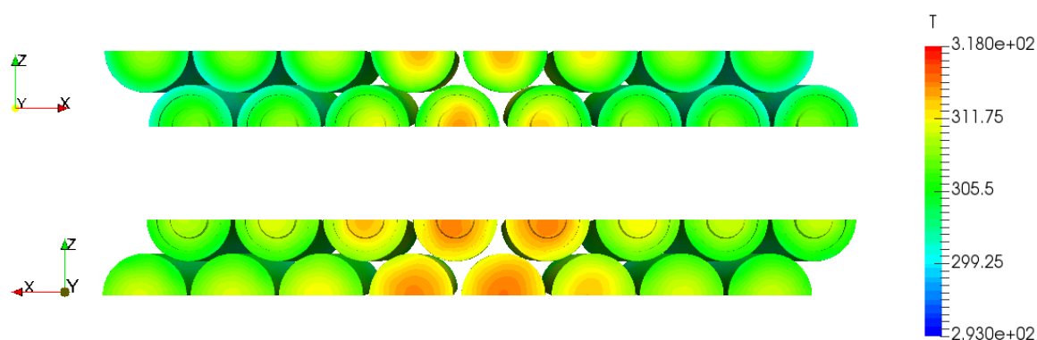
Slika 5.17 Temperaturno polje [K] ćelija pri brzini strujanja na ulazu od 20 m/s i neuniformnim razmakom između ćelija –strana ćelija bliže ulazima (gornja slika) i strana ćelija bliže izlazima (donja slika)
