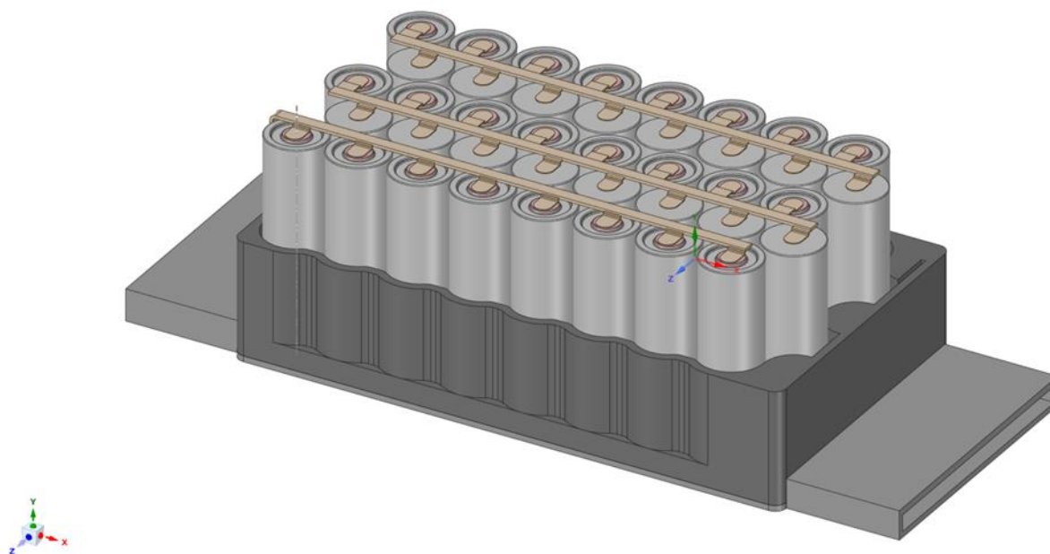
Slika 4.6 Dio kućišta modula s baterijama
