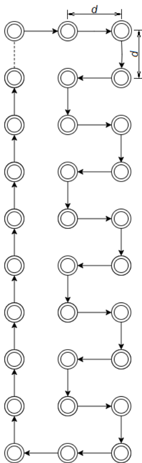
Slika 30. Putanja za jedno spajanje po prolazu
