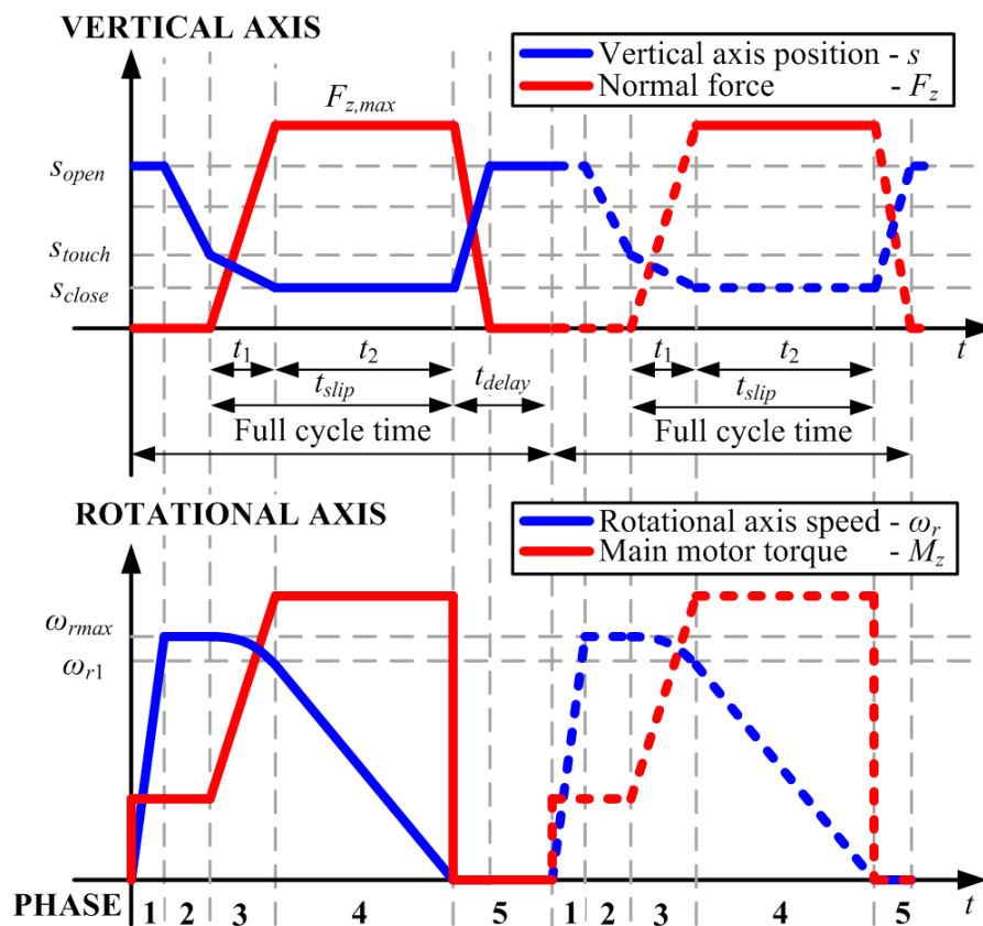
Slika 47. Kvalitativni prikaz faza radnog ciklusa ispitnog stroja ( [32])
