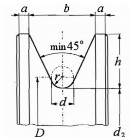
Slika 23. Profil užnice [1]
