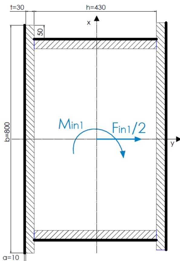
Slika 67. Opterećenje zavara uslijed sile inercije portala granika
