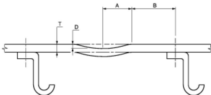
Slika 14. Parametri udubine [9]
