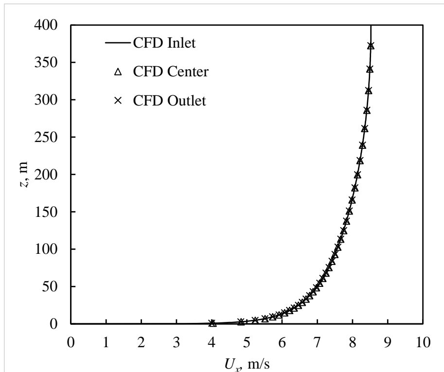
Slika 20 Usporedba profila brzine u 2D domeni s ulazim profilom prema Richardsu i Norrisu[22]
