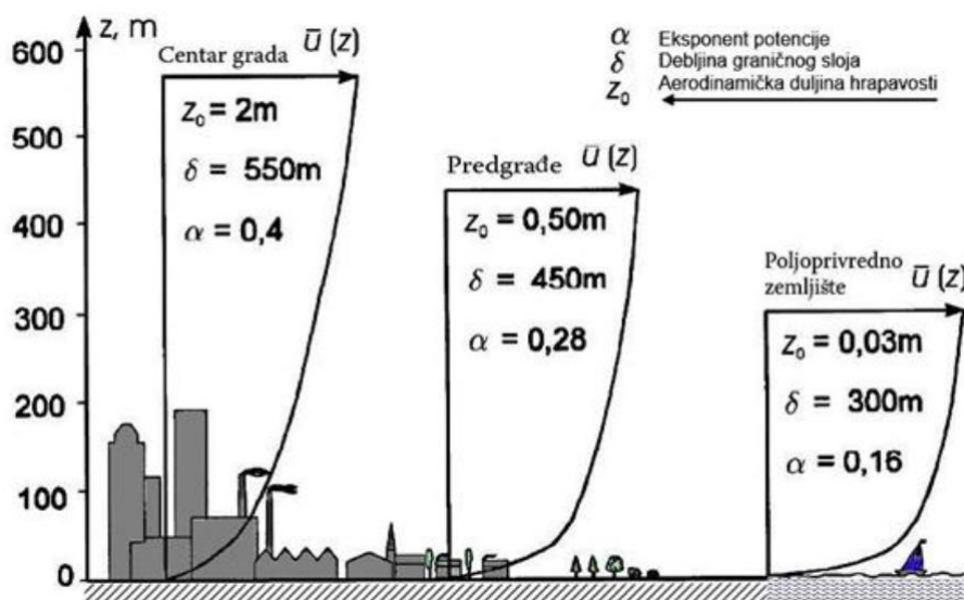
Slika 6 Profili homogenog atmosferskog graničnog sloja dobiveni zakonom potencije za strujanje nad tri različita tipa terena [29]
